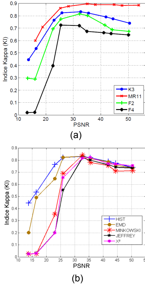
Figure 5 – (a) Indice KAPPA de la segmentation des quatre images testées en fonction du PSNR du bruit ajouté avant la LPE. (b) Indice Kappa de la segmentation de l'image F3 obtenue avec différentes mesures de dissimilarité en fonction du niveau de bruit ajouté avant LPE. De haut en bas : histogrammes cumulés, distance EMD (Earth Mover's Distance), distance de Minkowski, divergence de Jeffrey et distance \chi^2 .
